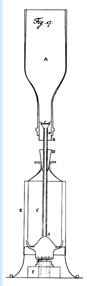
Nörrenbergs Kaffeemaschine (seine vielleicht wichtigste Erfindung!)
